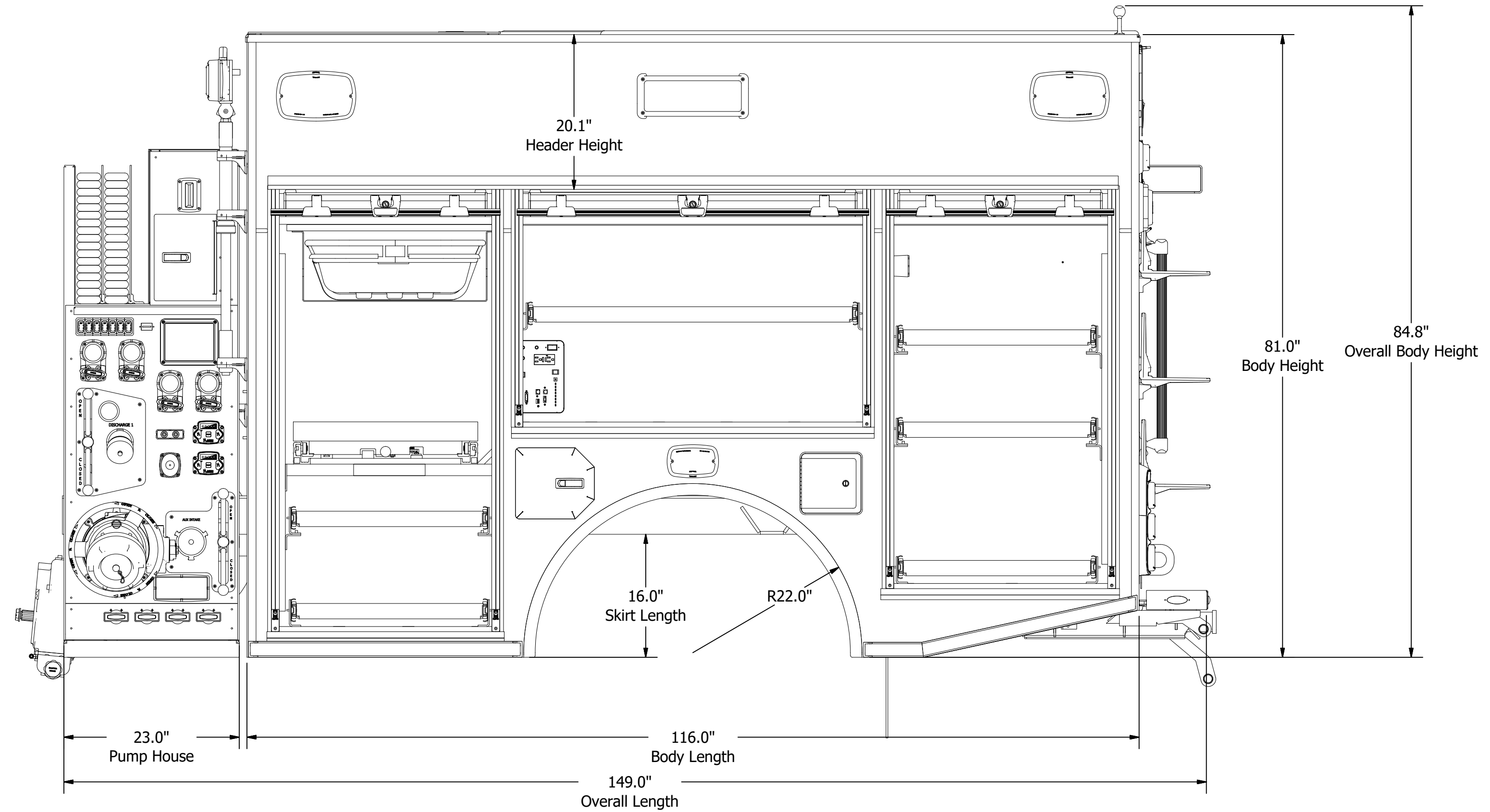
Body Dimensions
