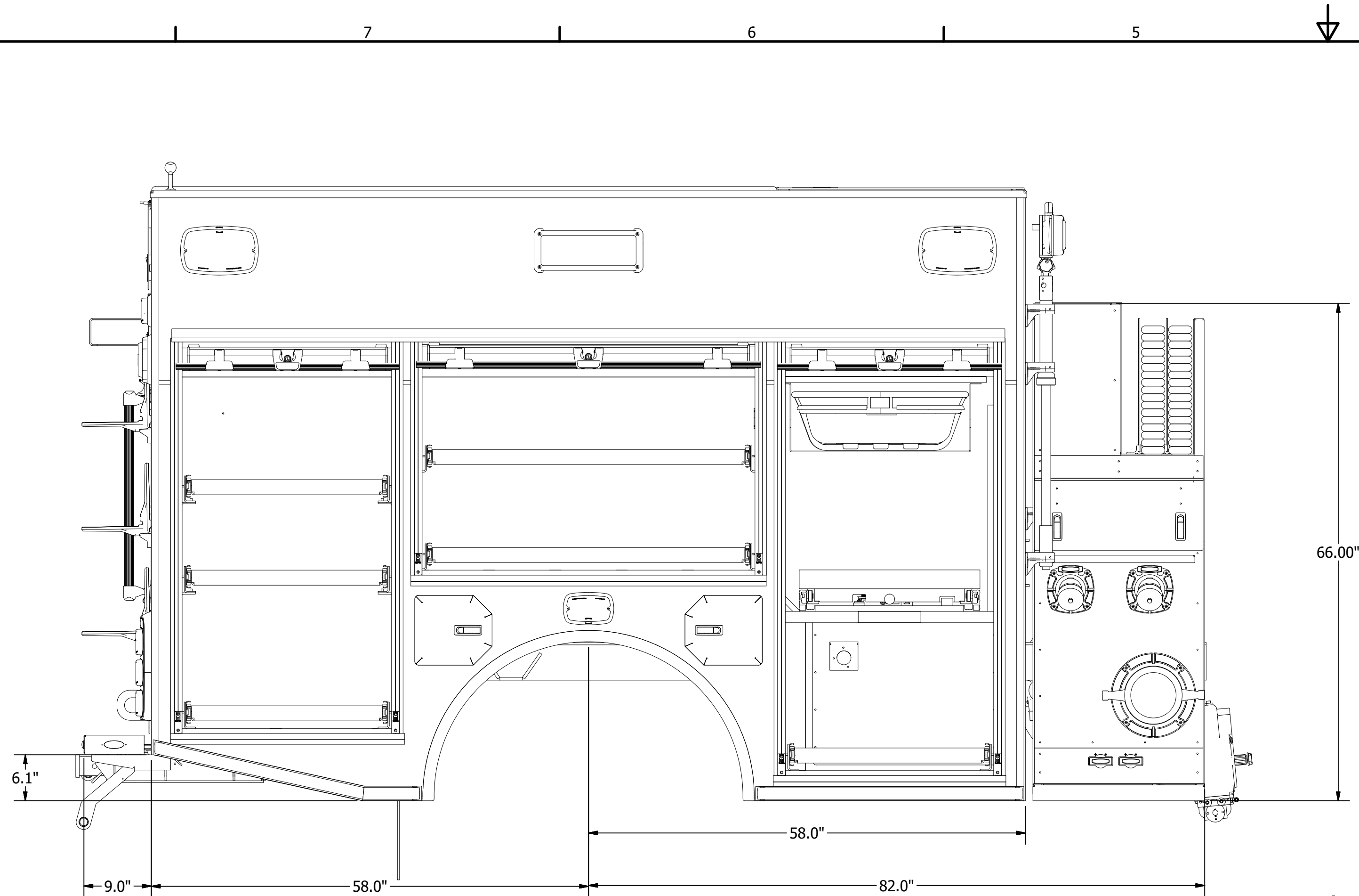
Body Dimensions
